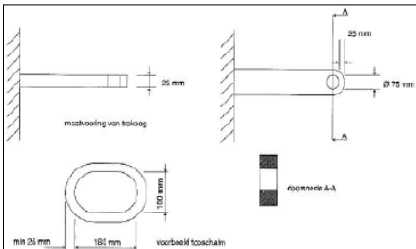
...organ... Figuur 2 Maatvoering trekhaak en topschalm
