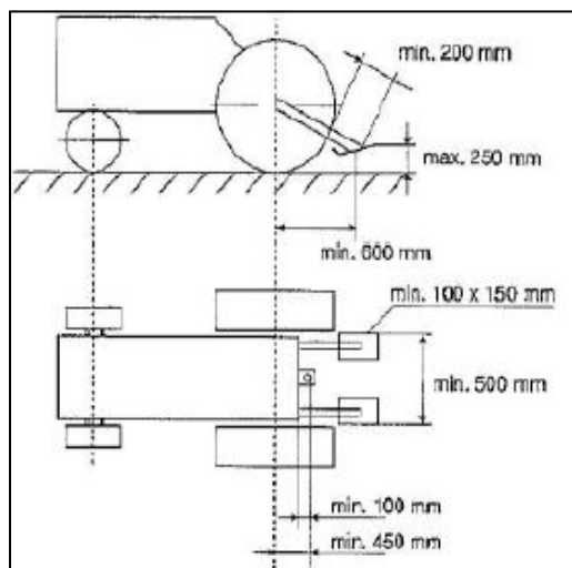
Verd... Figuur 1 Tekening steigerbegrenzer
